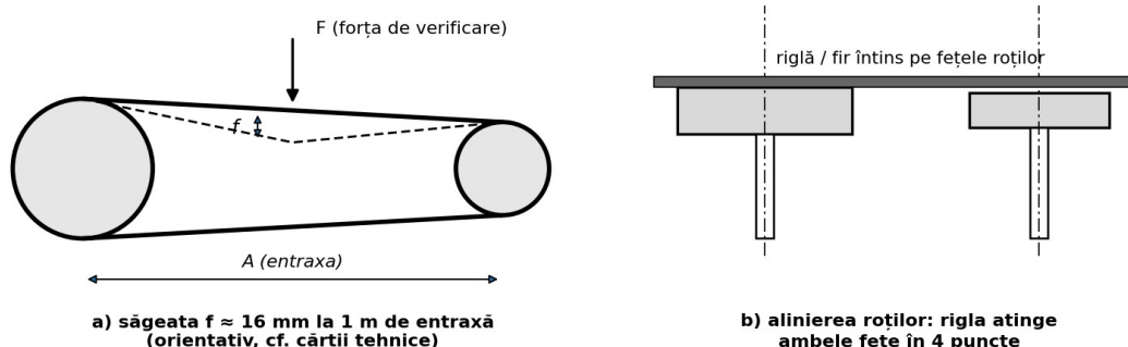
Fig. 12. Verificarea întinderii curelei prin săgeată și alinierea roților de curea (schematic)
