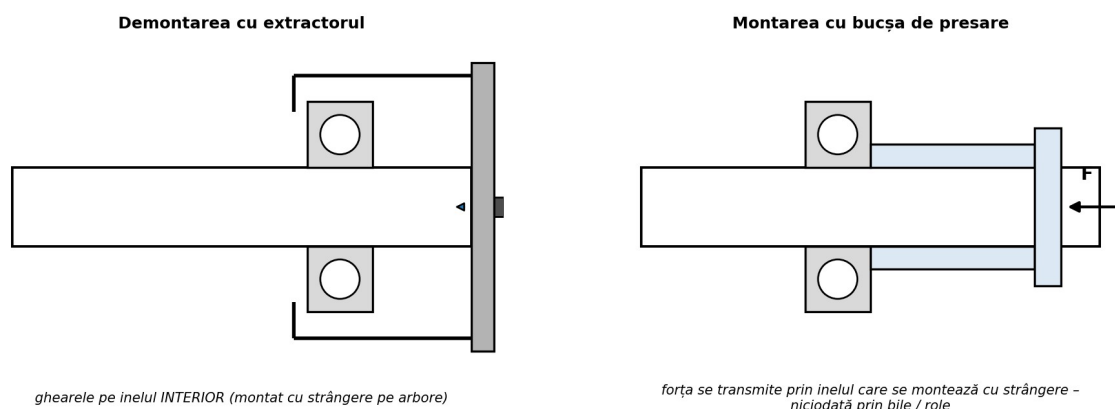
Fig. 17. Demontarea și montarea corectă a rulmentului: forța se aplică pe inelul montat cu strângere
