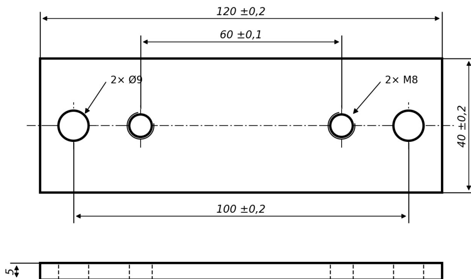
Fig. 6. Placa de fixare – desen de execuție
