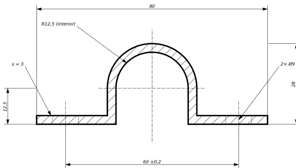
Fig. 7. Brida – desen de execuție (vedere frontală în secțiune)
