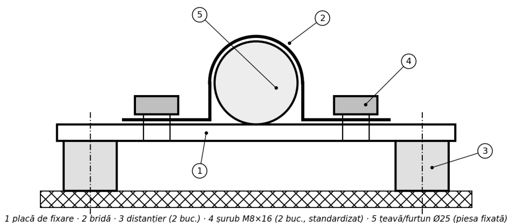
Fig. 9. Suportul de fixare cu bridă – desen de ansamblu (simplificat)
