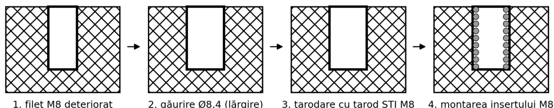
Fig. 12. Refacerea unui filet interior deteriorat cu insert filetat
