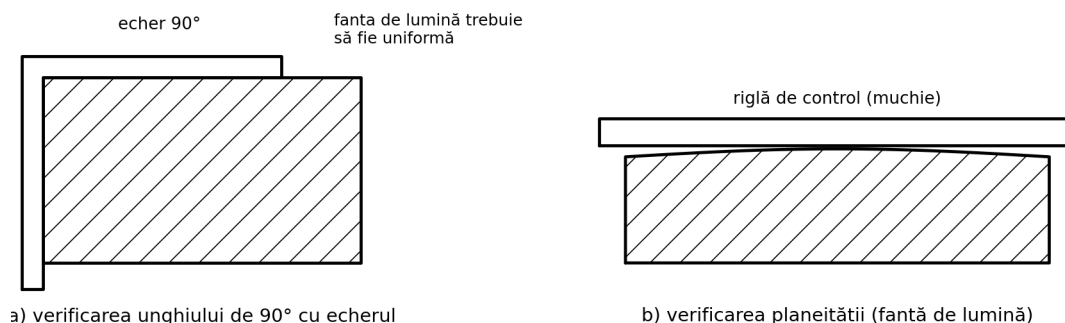
Fig. 9. Verificarea cu echerul (a) și cu rigla de control (b)
