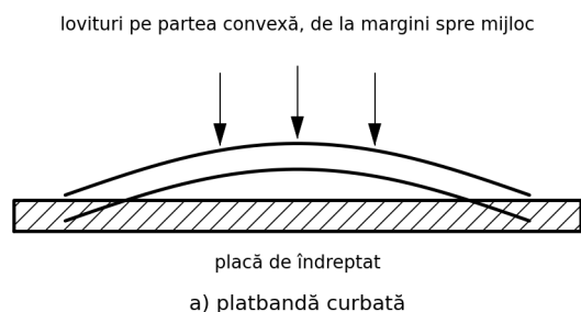
Fig. 10. Îndreptarea platbandei curbate și a tablei cu bombament
