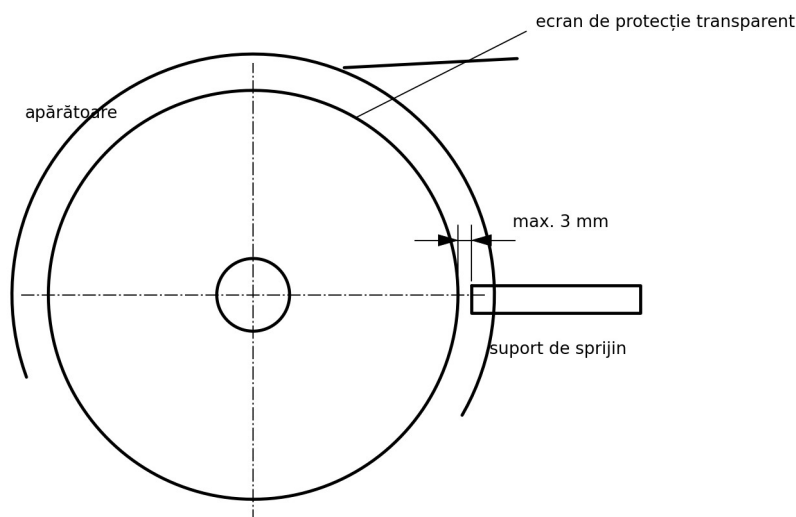
Fig. 19. Polizorul stabil: apărătoarea, ecranul și suportul la cel mult 3 mm
