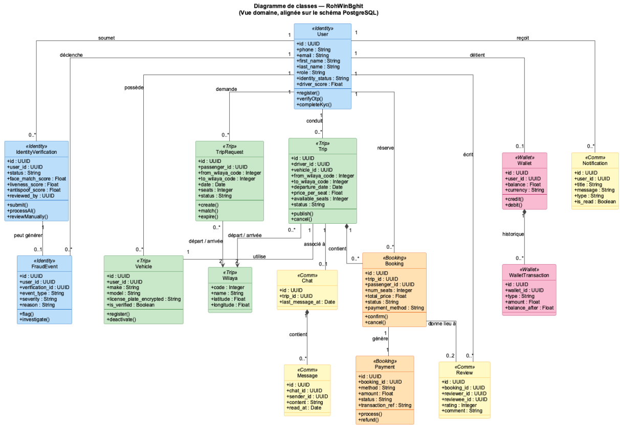
Fig. 2.2 – Diagramme de classes du domaine (alignement PostgreSQL)
