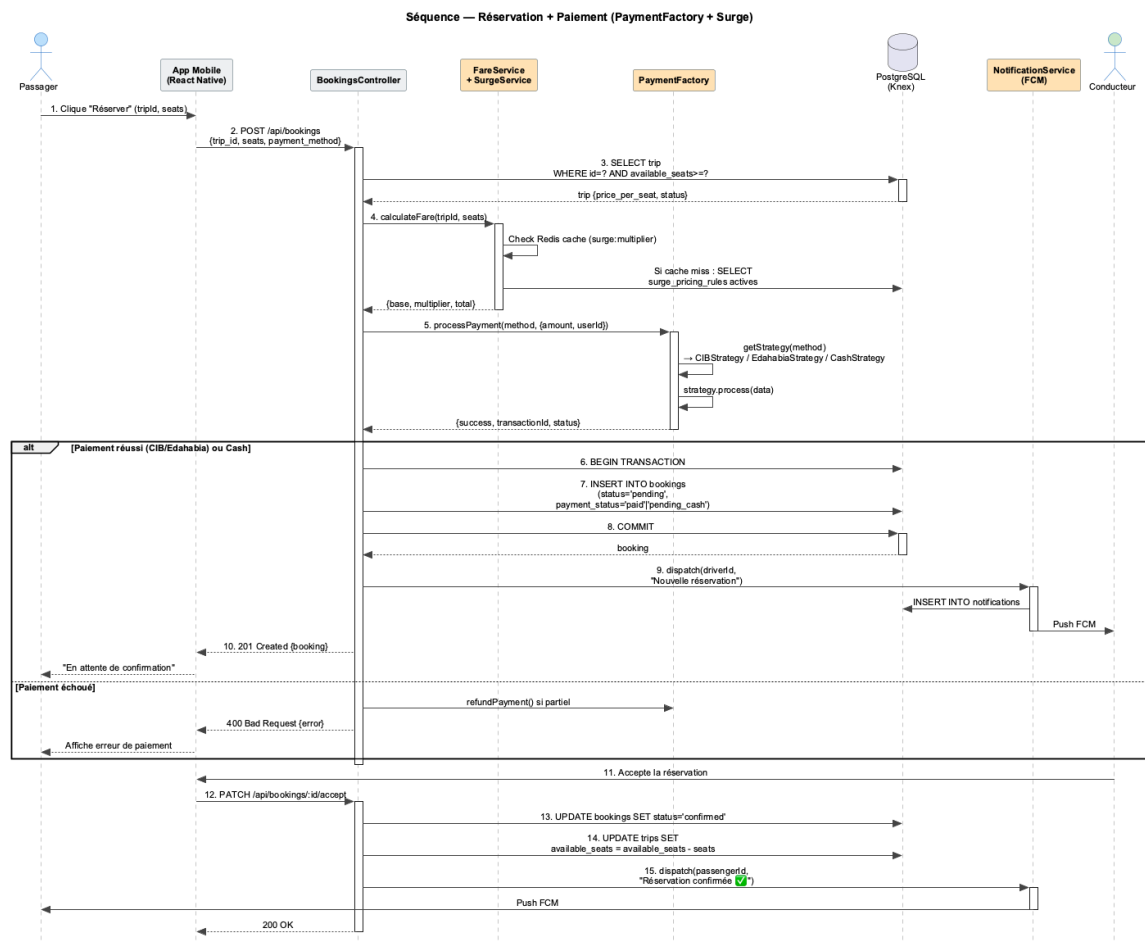
Fig. 2.3 — Séquence — Réservation avec paiement multi-méthodes (vue technique)
