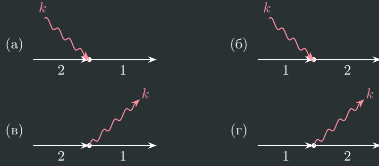
Диаграммы четырёх членов взаимодействия со слайда. Прямая линия — атом, волнистая — фотон, вершина — одно действие взаимодействия. Время направлено слева направо.
