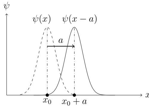
Рис. 1: Активное преобразование: волновая функция смещается в фиксированной системе координат. Исходная функция \psi(x) (штриховая линия) преобразуется в \psi(x-a) (сплошная линия) согласно \hat{T}_a\psi(x) = \psi(x-a) .
