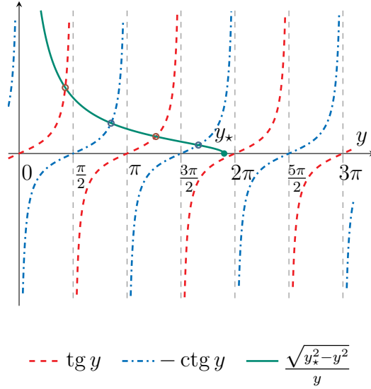
Рис. 5: Графическое решение уравнений для уровней энергии в прямоугольной яме. Чётные уровни энергии соответствуют точкам пересечения кривой \text{tg } y с функцией \sqrt{y_*^2 - y^2}/y (красные точки), а нечётные — точкам пересечения -\text{ctg } y с той же функцией (синие точки).
