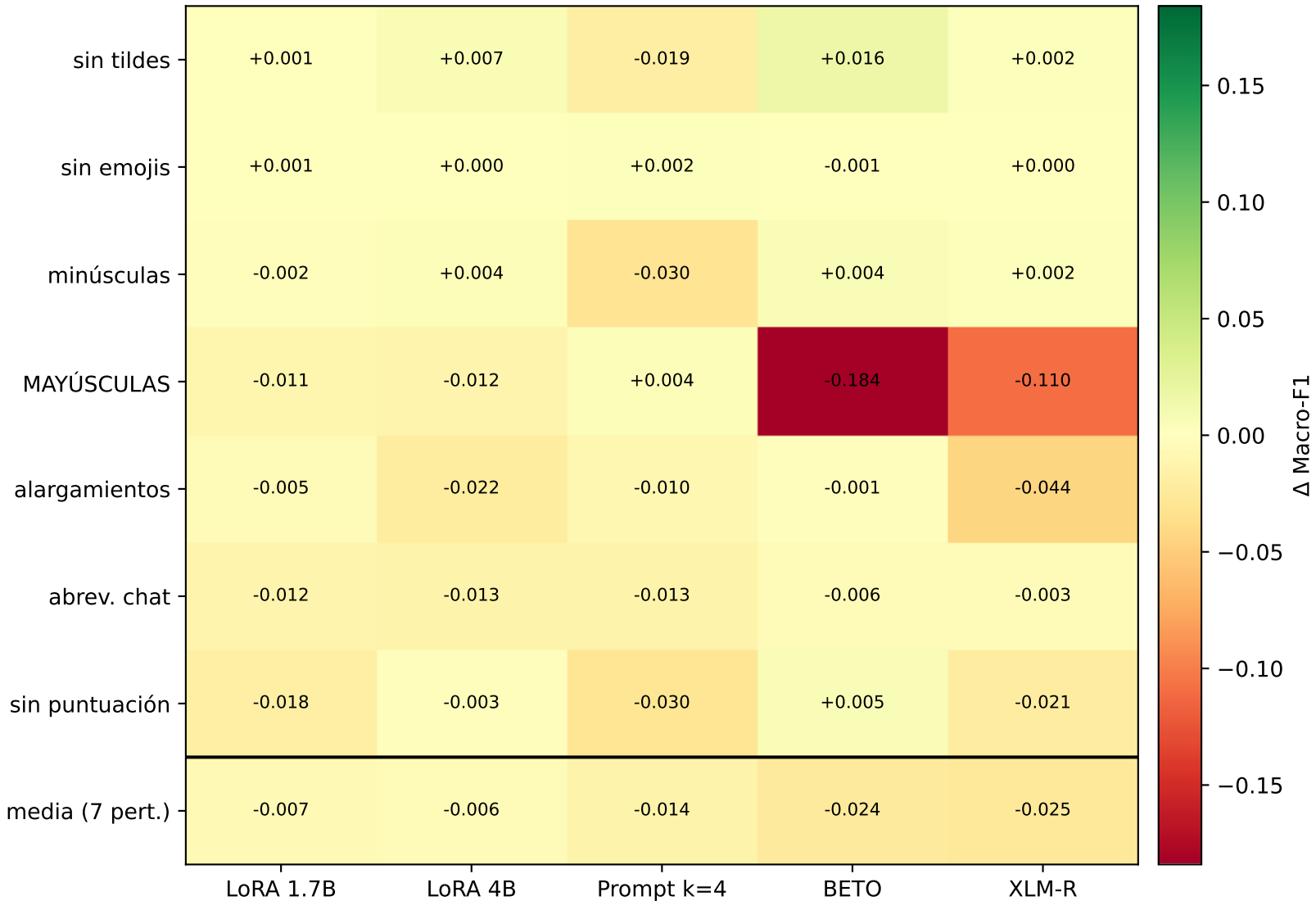
Robustez al ruido del español de redes (re-inferencia, pesos congelados) \Delta Macro-F1 vs limpio (perturbado – limpio) — rojo = se degrada Test Cardiff ES (n=870, semilla 42). Fuente: results/robustness_results.csv
