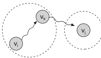
Camino de v_i - v_k - v_j
