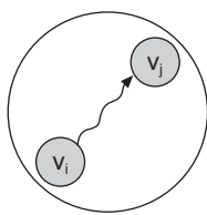
Camino de v_i a v_j
