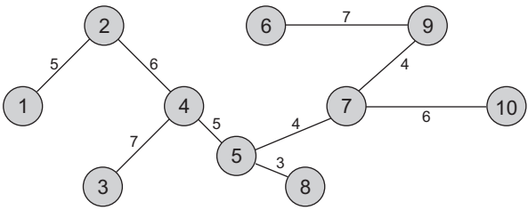
Figura 18.26. Árbol de expansión del grafo de la Figura 18.25.
