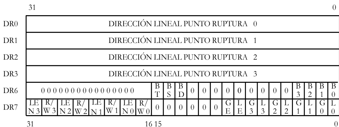
Figura 11.13. Formato de los seis registros de depuración que tienen definidas funciones en el Pentium.
