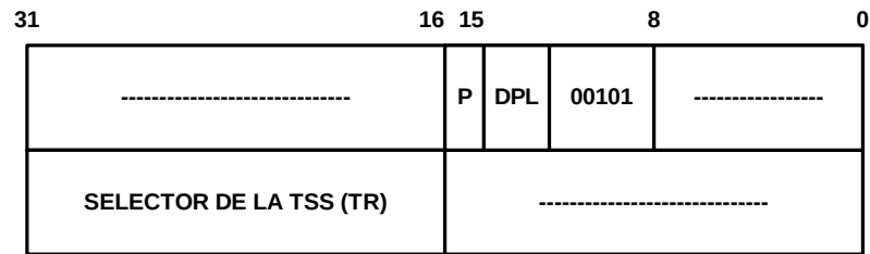
Figura 14.11 – Puerta de Tarea.
