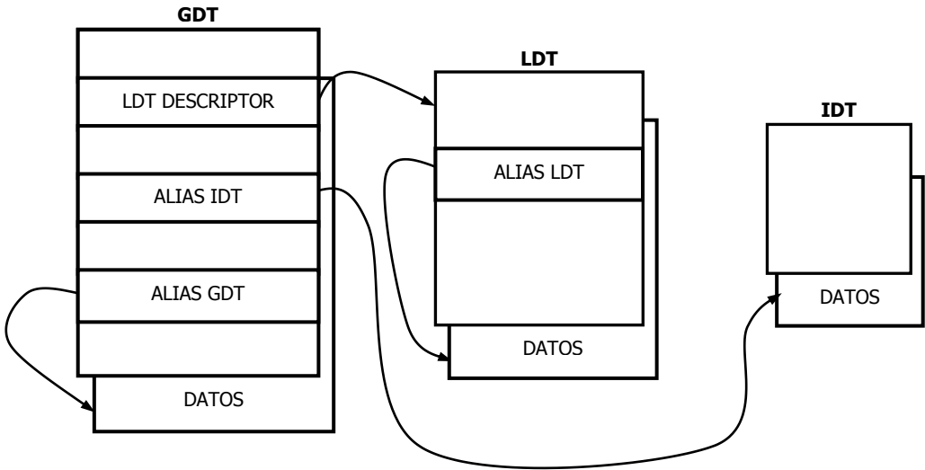
Figura 12.19. Los descriptors alias en la GDT son siempre accesibles.
