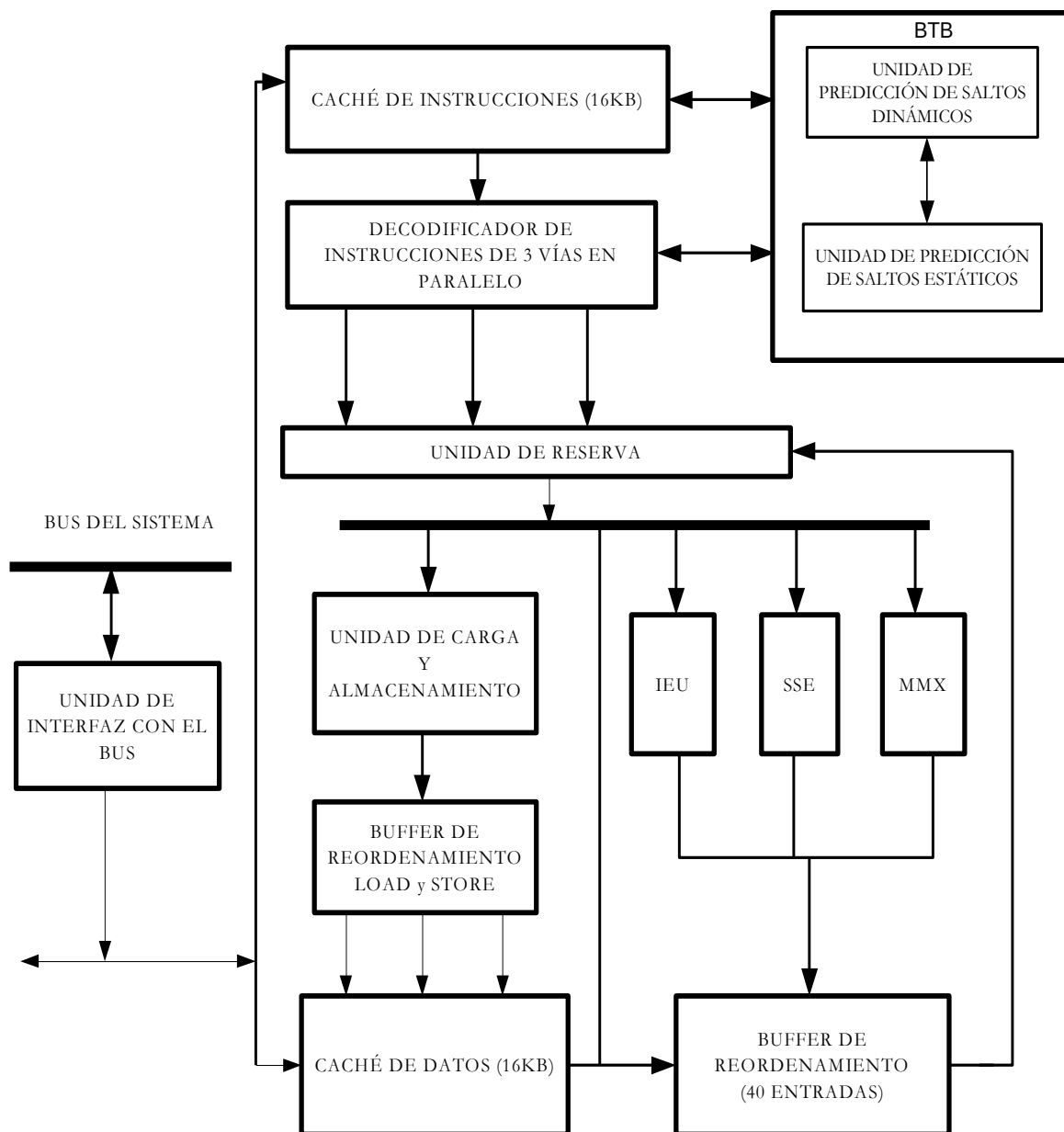
Figura 23.1 – Arquitectura del Pentium III
