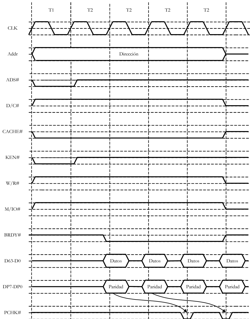
Figura 27 - Ciclo de bus a ráfagas
