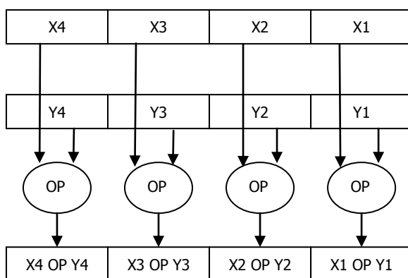
Figura 25.3. Esquema de operación SIMD.
