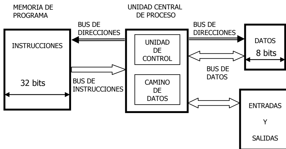
Figura 1.11. Arquitectura Harvard.
