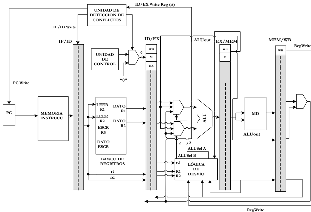
Figura 48.- Actuación de la Unidad de Detección de conflictos cuando trata los precedentes de las dependencias de datos con instrucciones de transferencia con memoria.
