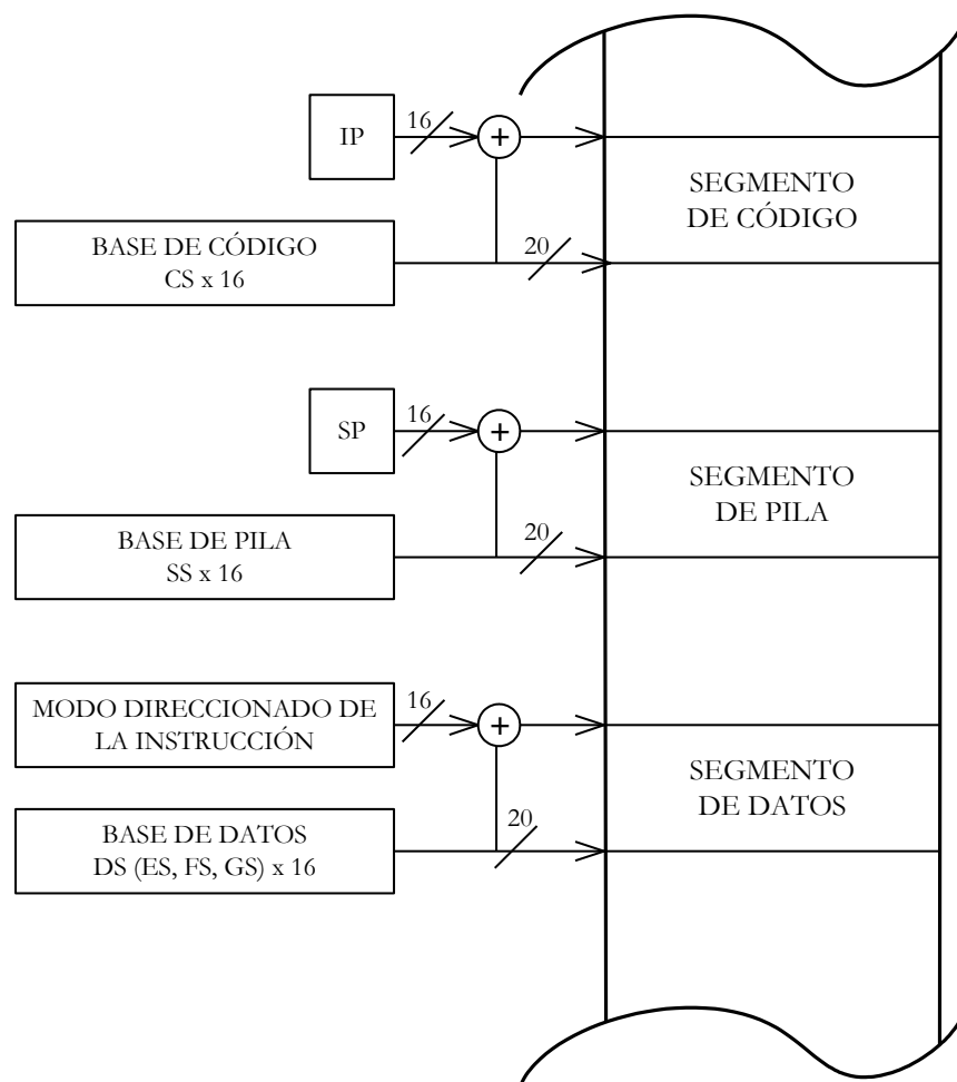
Figura 7.13 – Segmentación en modo real. En este modo se accede a elementos de memoria multiplicando por 16 el valor del registro de segmento y añadiendo un desplazamiento de 16 bits al resultado.
