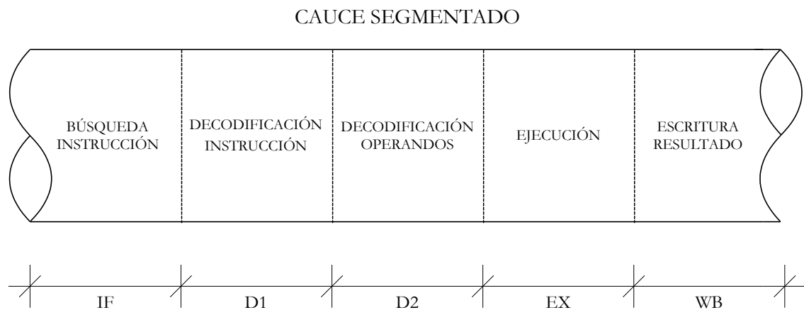
Figura 6.5 – Etapas del cauce segmentado
