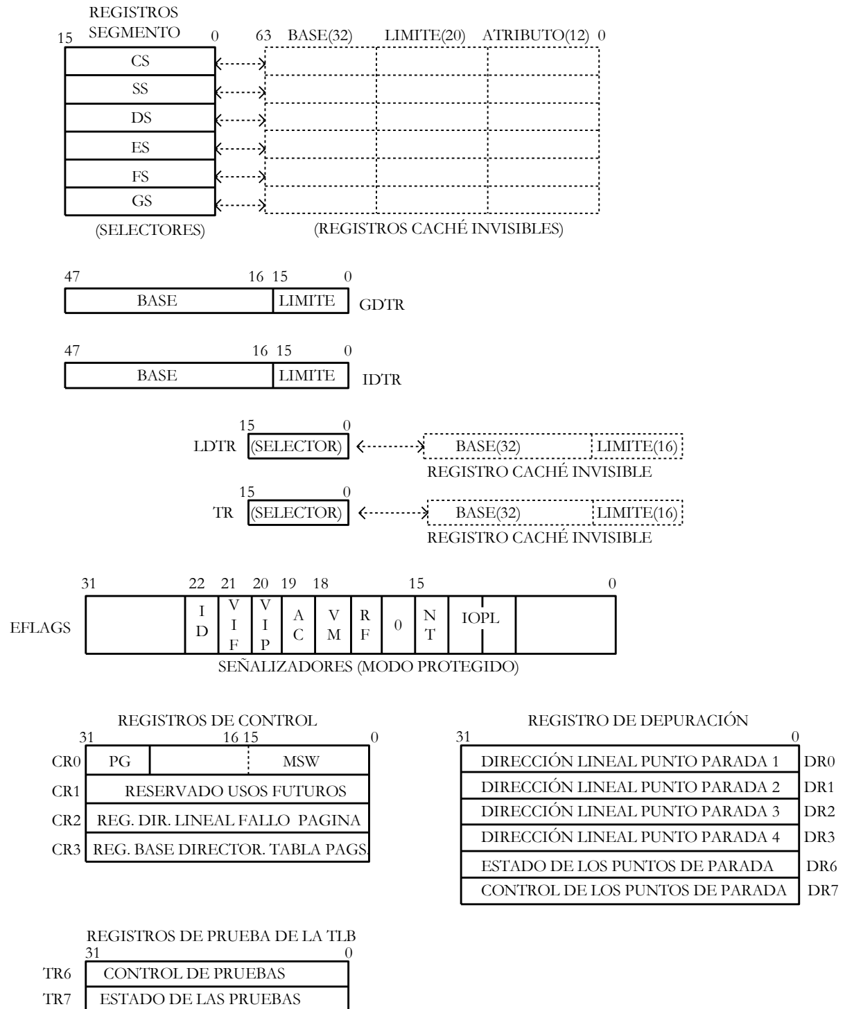
Fig. 11.1. Registros del sistema.
