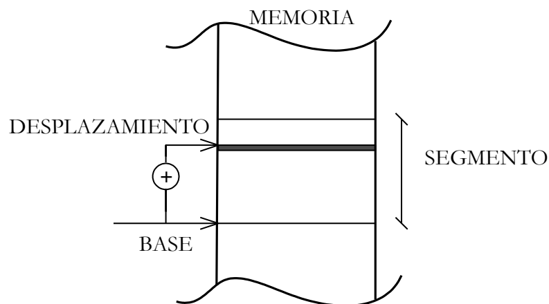
Figura 7.11 – Dirección lógica de un elemento (desplazamiento)
