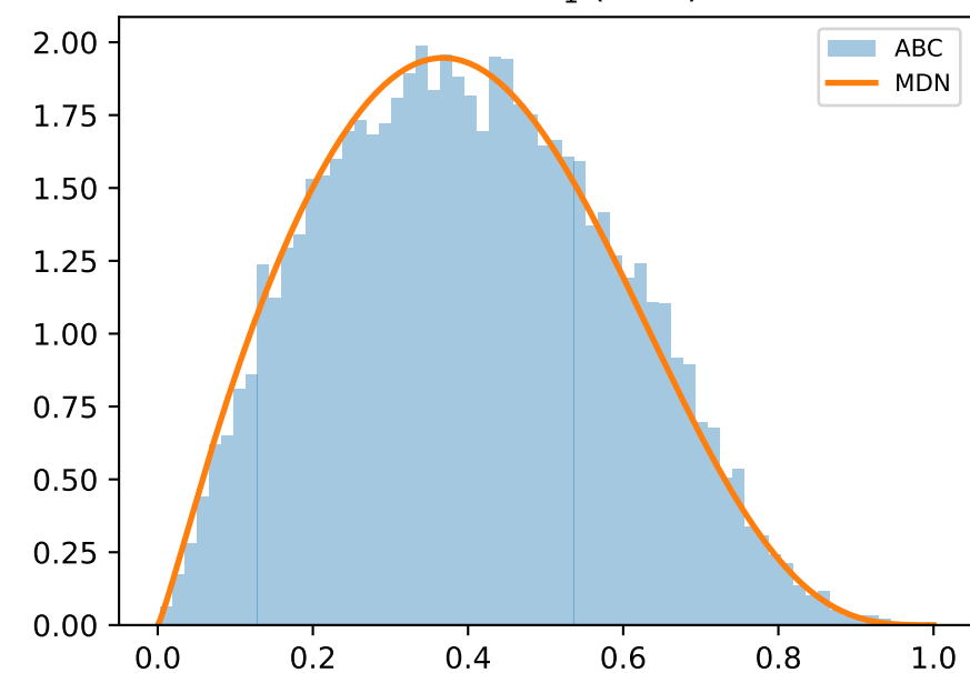
x=0.21 \theta_1 (Beta)
