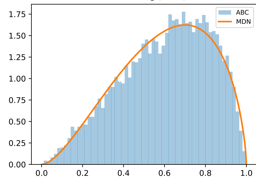
x=0.93 \theta_1 (Beta)
