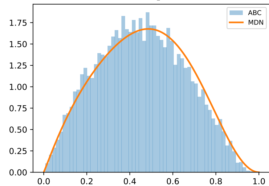
x=-0.73 \theta_1 (Beta)
