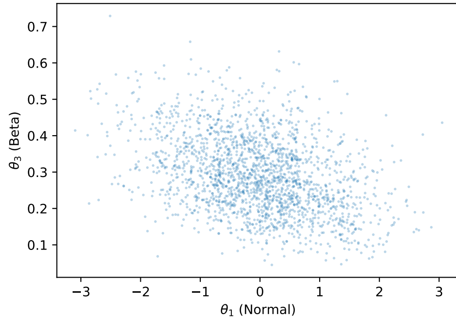
ABC posterior x_obs=5.31
