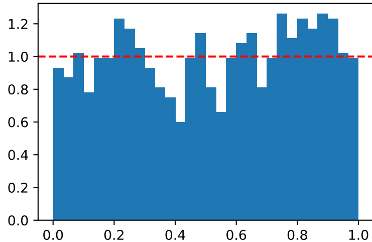
PIT t3 (Beta)
