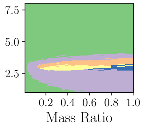
e = 0.8
