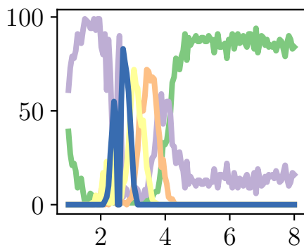
e = 0.8
