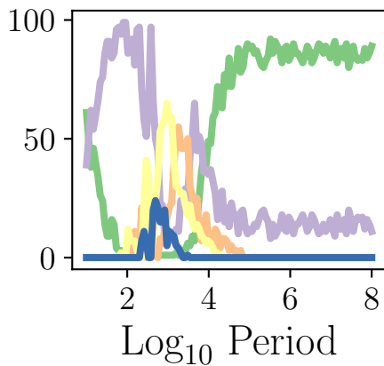
e = 0.8
