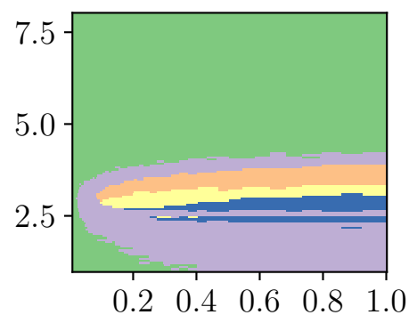
e = 0.8
