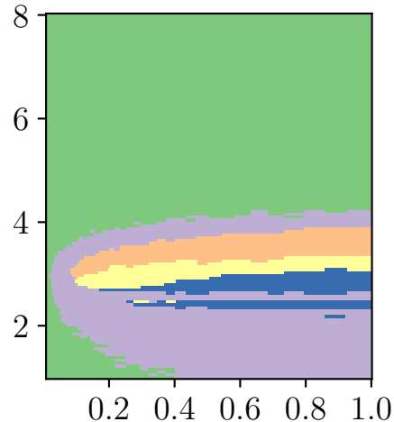
e \equiv 0.8
