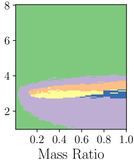
e \equiv 0.8
