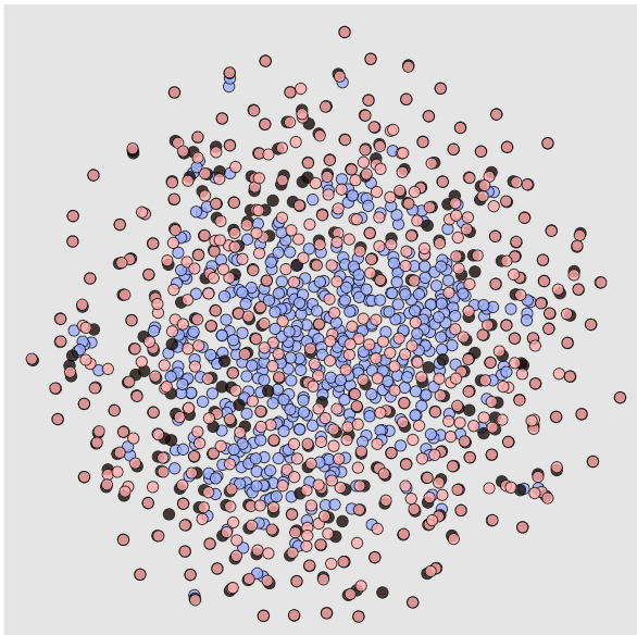
Raw
