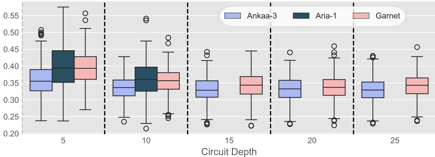
JS-divergence
