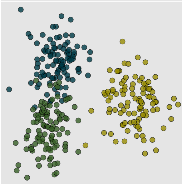
Log Ratio (Var: 0.234)
