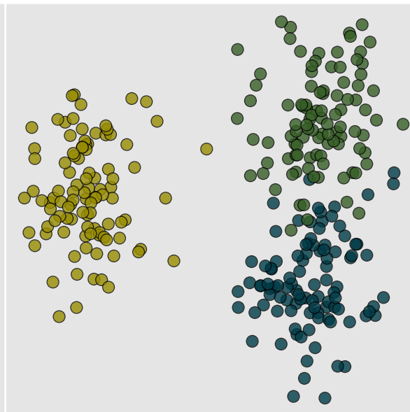
Residual (Absolute) (Var: 0.286)
