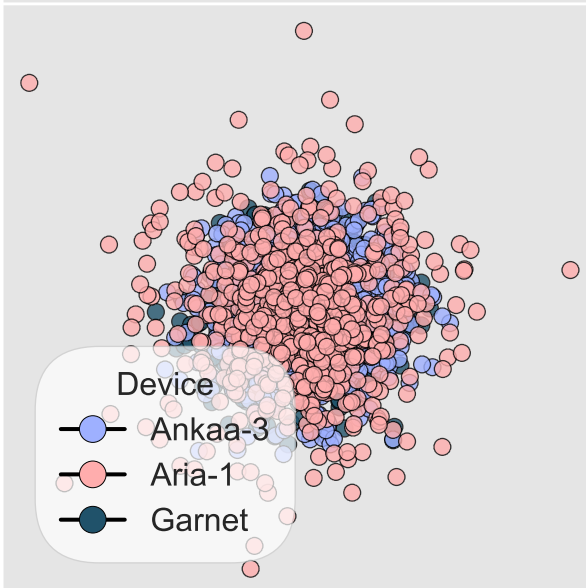
Log Ratio (Var: 0.096)
