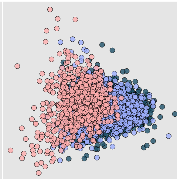
Residual (Absolute) (Var: 0.089)
