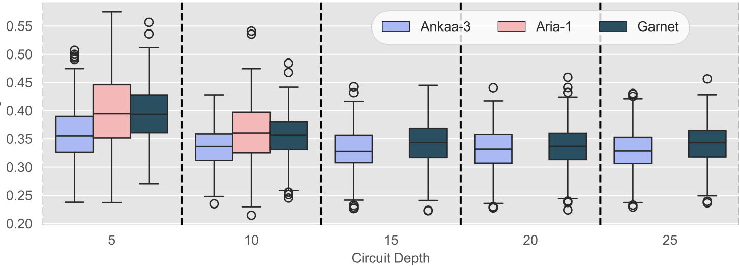
JS-divergence
