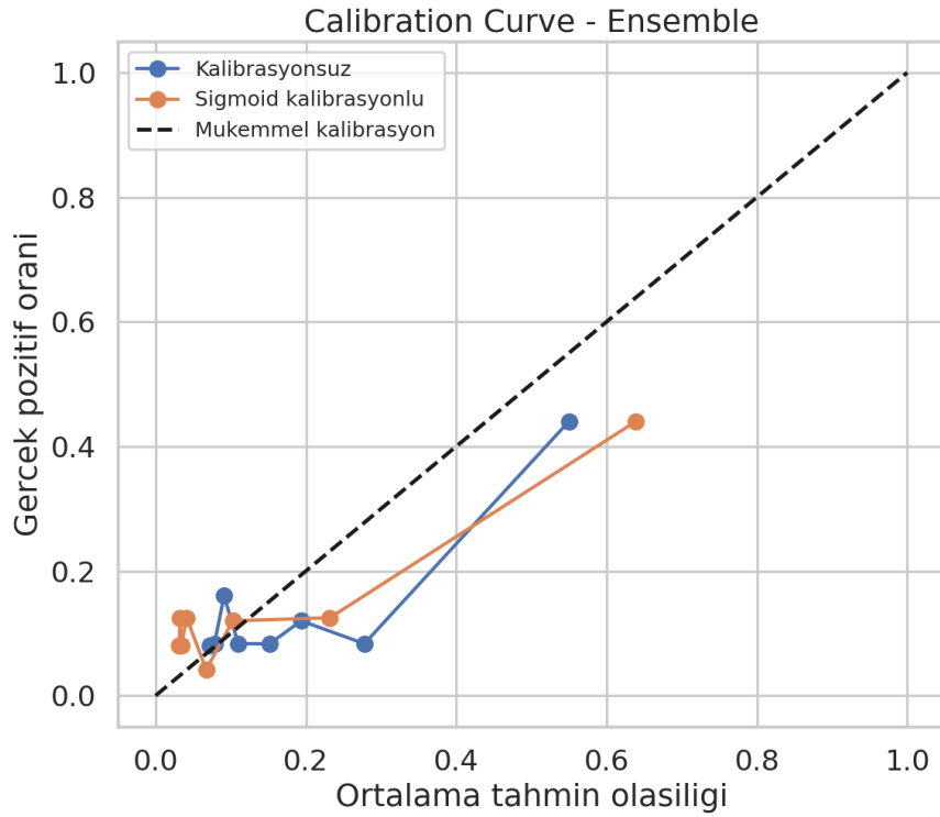
Şekil 6. Ensemble için kalibrasyon eğrisi (sigmoid kalibrasyon öncesi/sonrası).
