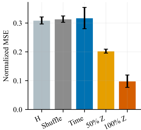
ETTh1
