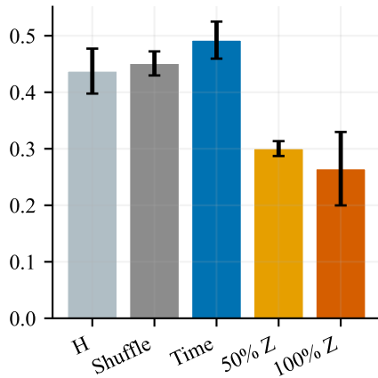
ETTh2
