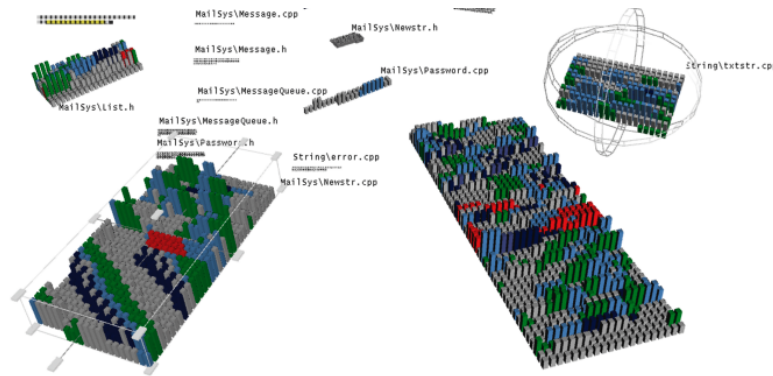
Abbildung 5.5: 3D Pixel Bars: Für jede Datei gibt es eine eigene Visualisierung auf Zeilenebene [MFM03, S. 7].
