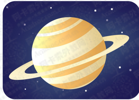
planet
