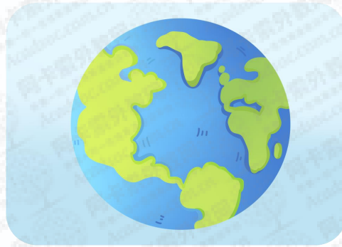
earth
