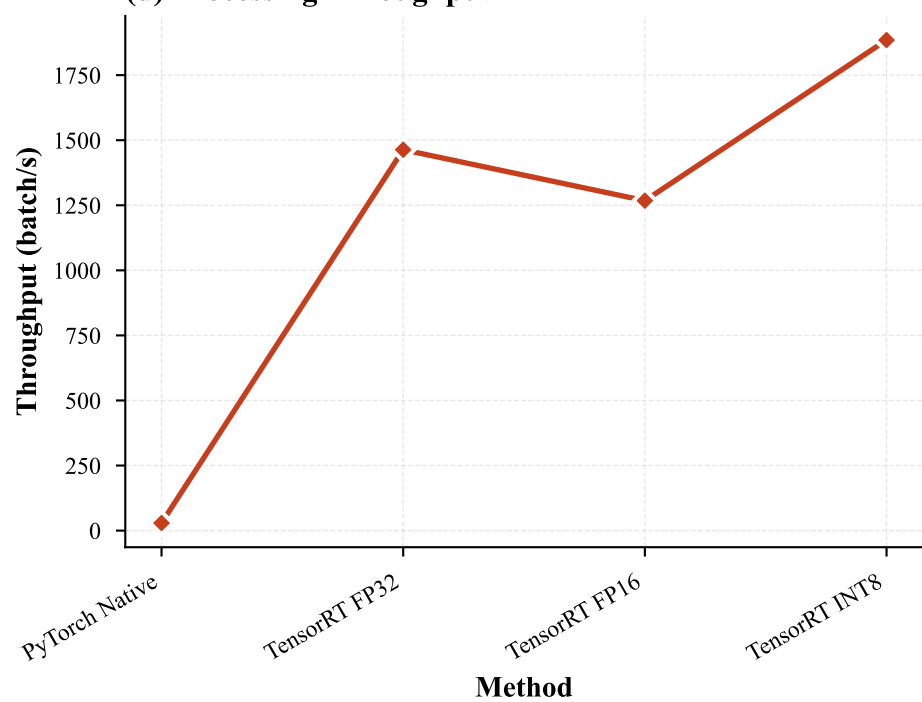
(d) Processing Throughput
