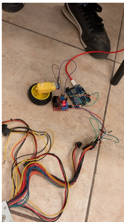
Figura 2. Vista del motor con rueda, la placa Arduino y el cableado del montaje.
