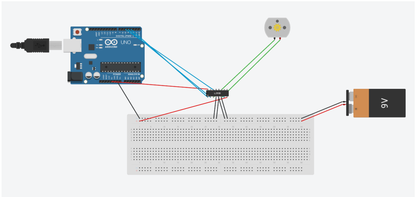
Figura 1. Esquema de referencia del motor y el puente H. El dibujo muestra una batería de 9 V; el reporte describe una fuente externa de 12 V para el montaje físico.
