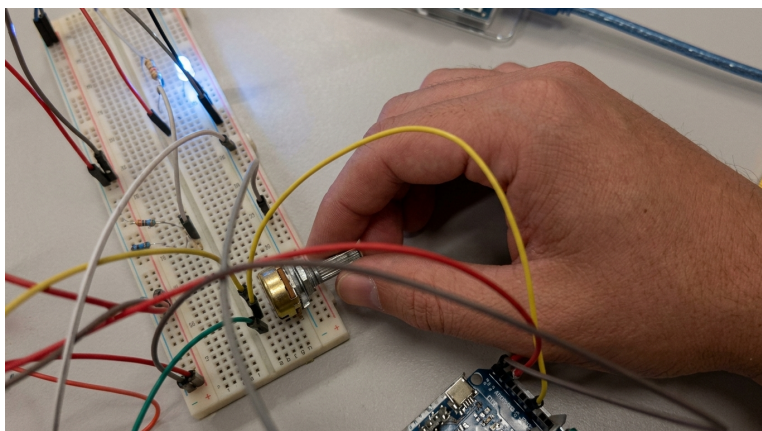
Figura 3. Detalle del ajuste del potenciómetro (Esclavo 3) y su efecto en tiempo real sobre el ángulo del servomotor.
