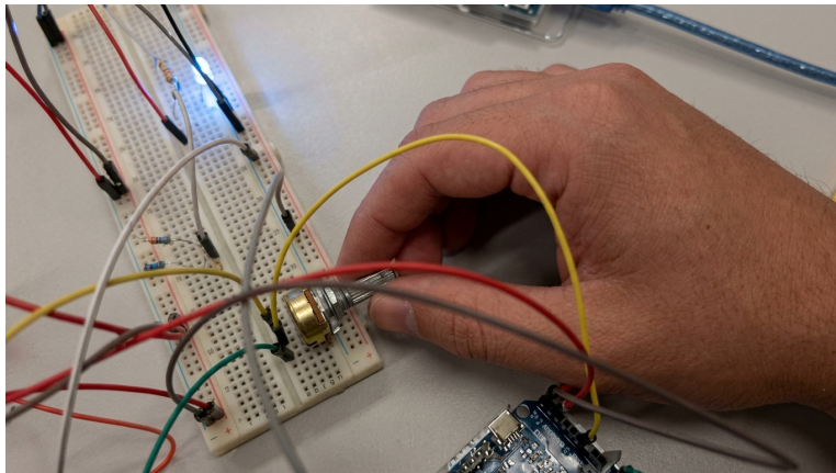
Figura 2. Detalle del potenciómetro (Esclavo 3) siendo ajustado para controlar el ángulo del servomotor.
