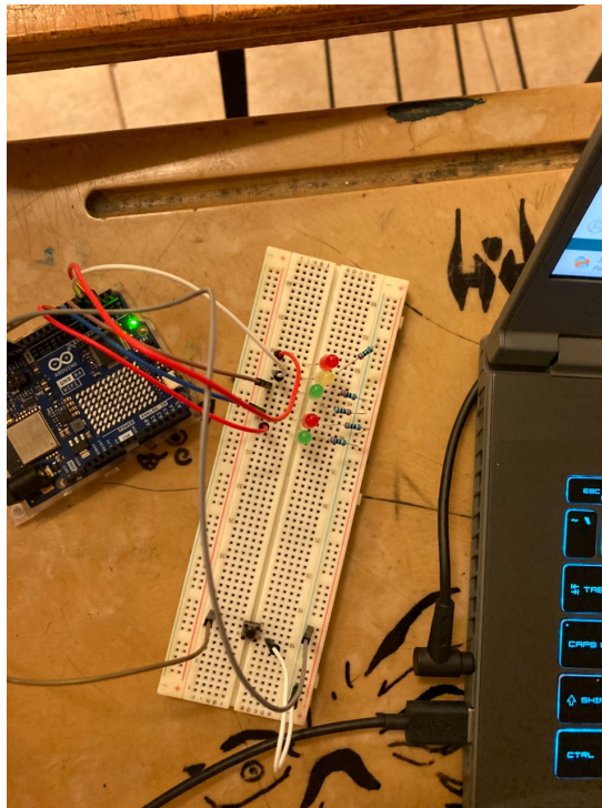
Figura 2. Montaje de los LEDs y del pulsador en la protoboard.
