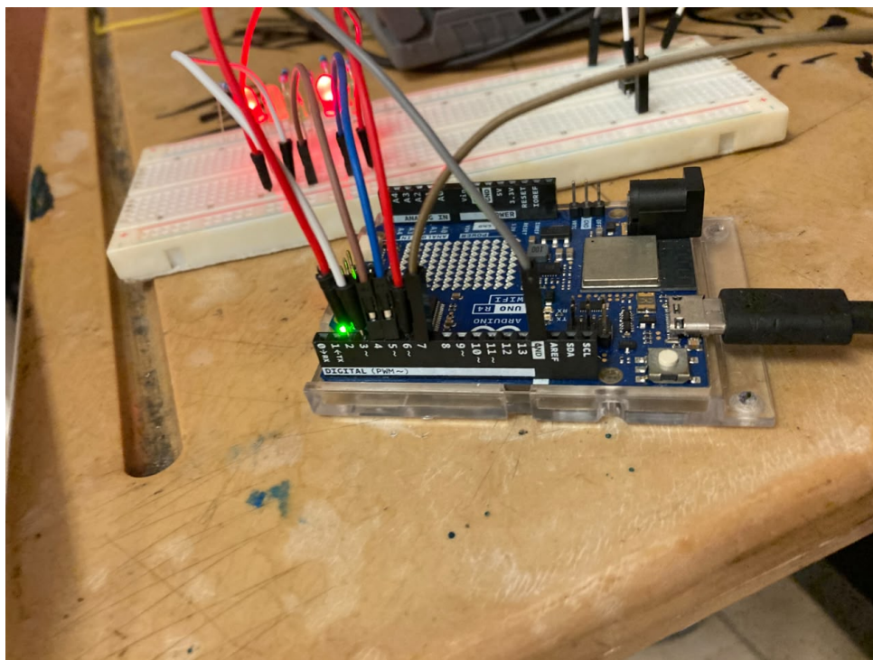
Figura 3. Detalle de las conexiones entre la placa Arduino y la protoboard.
