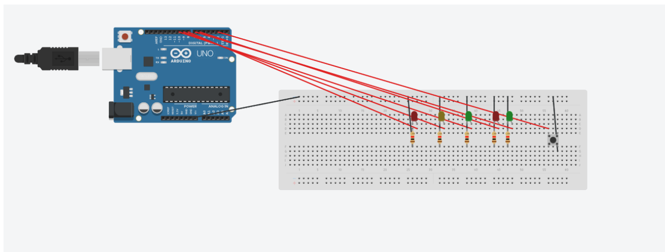
Figura 1. Diagrama del semáforo: LEDs vehiculares, LEDs peatonales y pulsador de solicitud de cruce.
