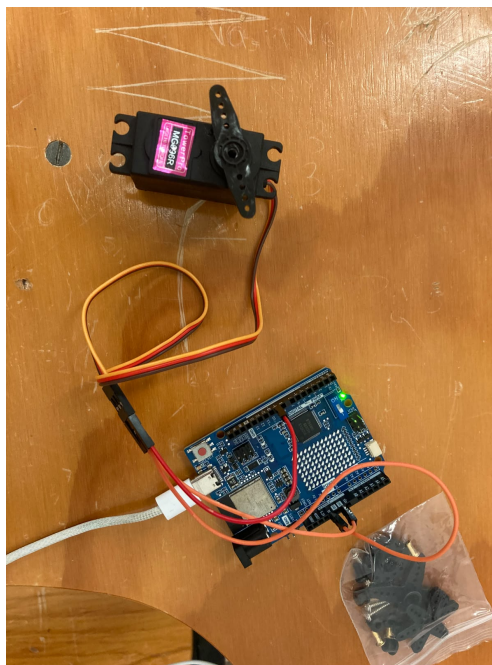
Figura 2. Montaje físico del servomotor conectado a la placa Arduino UNO R4 WiFi.
