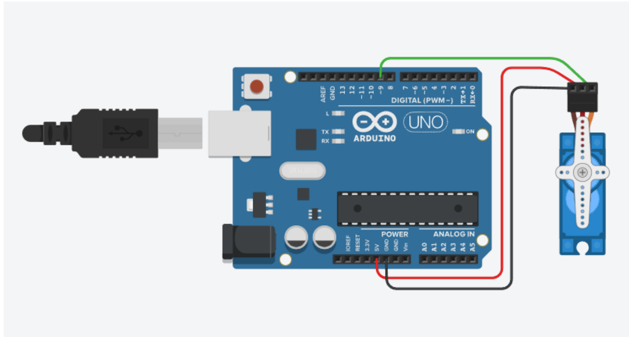
Figura 1. Diagrama de referencia de las conexiones de señal, alimentación y tierra del servomotor.
