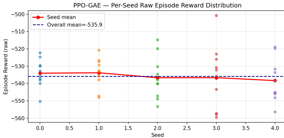
Figura 10: Distribución del reward de PPO-GAE sobre 5 semillas \times 20 episodios.
