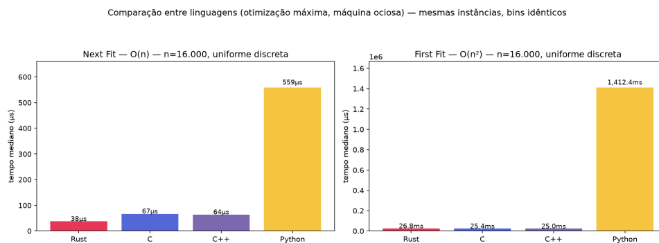
Figura 2. Tempo mediano por linguagem e algoritmo ( n = 16,000 , uniforme discreta). Compilados (Rust, C, C++) convergem nos quadráticos; Python fica \approx 15\text{--}63\times atrás.
