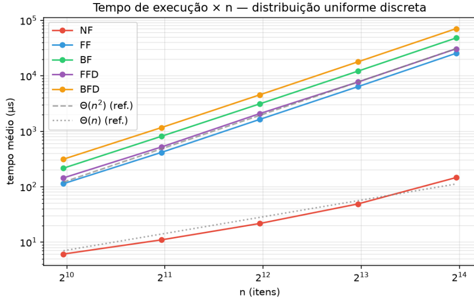
Figura 3. Tempo de execução em função do tamanho da instância ( n ), em escala log-log. O slope das curvas confirma a complexidade linear de NF ( \approx 1 ) e quadrática de FF/BF ( \approx 2 ), validando a previsão assintótica.
