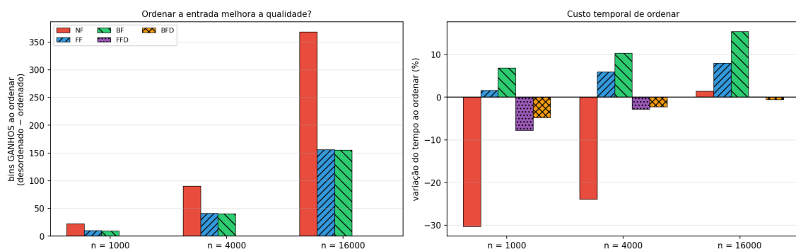
Figura 3. Efeito de ordenar a entrada, medido sobre a distribuição 3-partição (10 repetições por ponto). Esquerda: bins economizados ao ordenar (desordenado — ordenado); valores positivos indicam que ordenar ajudou. Direita: variação percentual do tempo de execução causada pela ordenação. Para FFD e BFD a economia é exatamente zero, pois a ordenação é parte da definição do algoritmo — as barras respective ficam na linha zero.
