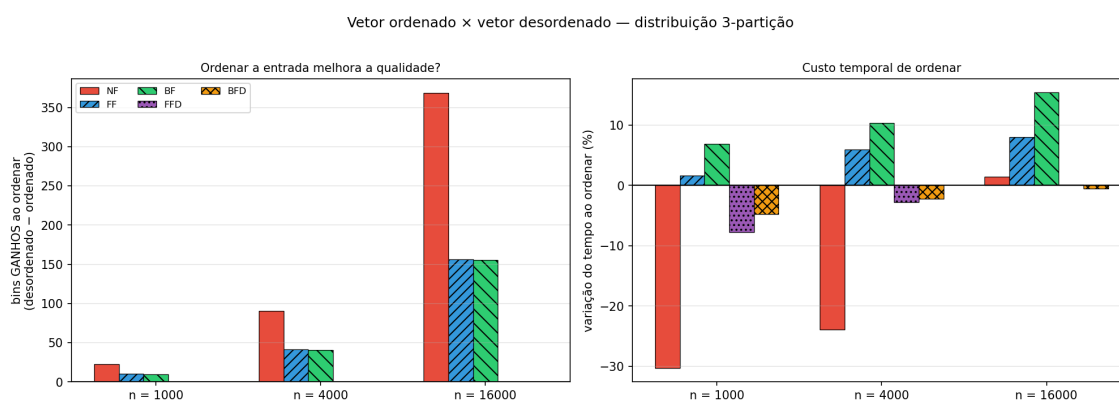
Figura 3. Efeito de ordenar a entrada, medido sobre a distribuição 3-partição (10 repetições por ponto). Esquerda: bins economizados ao ordenar (desordenado – ordenado); valores positivos indicam que ordenar ajudou. Direita: variação percentual do tempo de execução causada pela ordenação. Para FFD e BFD a economia é exatamente zero, pois a ordenação é parte da definição do algoritmo — as barras respective ficam na linha zero.
