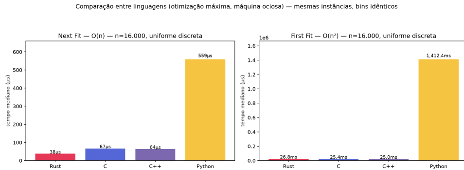
Figura 5. Tempo mediano por linguagem e algoritmo ( n = 16,000 , uniforme discreta). Compilados (Rust, C, C++) convergem nos quadráticos; Python fica \approx 15 – 63\times atrás.
