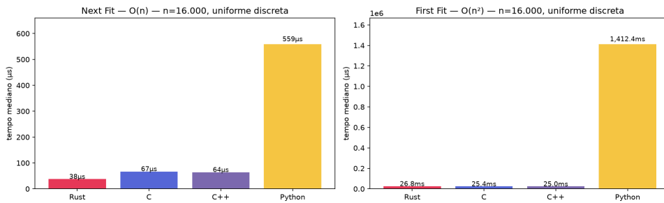
Figura 5. Tempo mediano por linguagem e algoritmo ( n = 16,000 , uniforme discreta). Compilados (Rust, C, C++) convergem nos quadráticos; Python fica \approx 10 – 61\times atrás.
