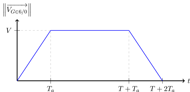
FIGURE 4 – Cycle en trapèze de la loi de commande de l'actionneur
