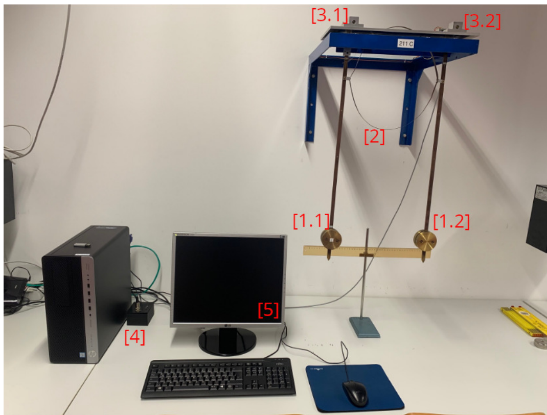
Abb. 1.2: Versuchsaufbau/Geräte 1
