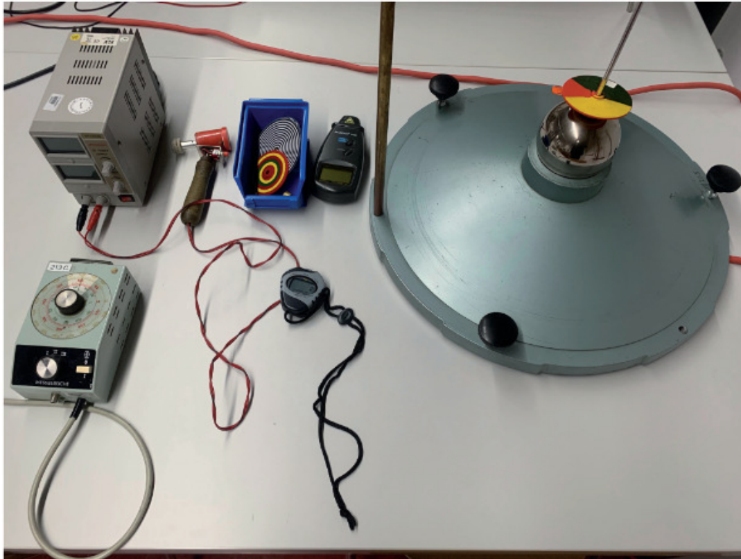
Abb. 1.1: Versuchsaufbau/Geräte 3
