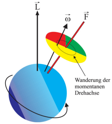
Abb. 1.3: Farbscheibe zur Bestimmung von \Omega 3
