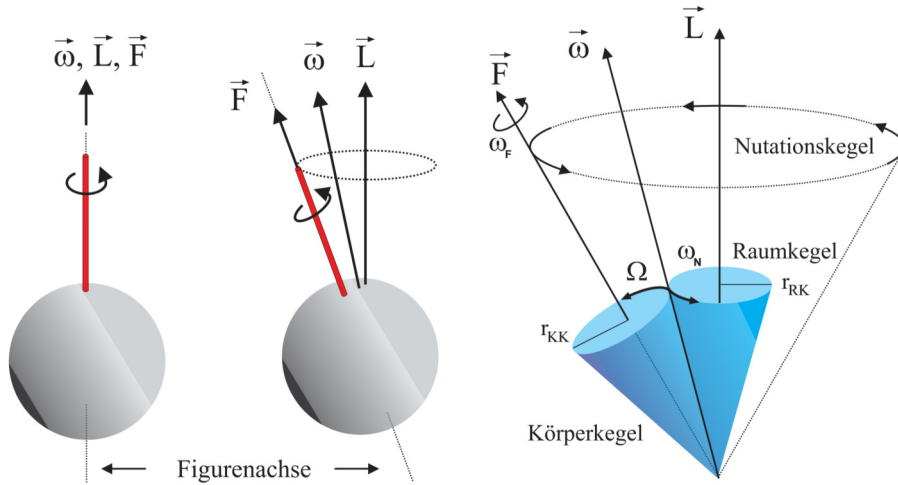
Abb. 1.2: Links: kräftefreier, symmetrischer Kreisel. Rechts: Nutationsbewegung selbigen Kessels nach einem Stoß: Achsen nicht mehr identisch und Körperkegel rollt auf Raumkegel ab 3
