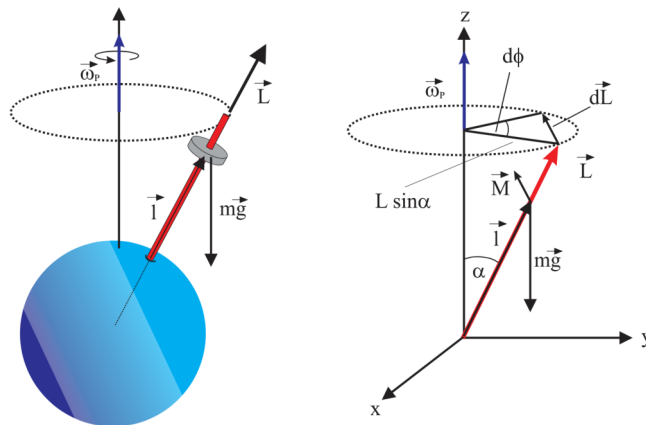
Abb. 1.4: Darstellung und Geometrie des schweren symmetrischen Kreisels zur Bestimmung der Präzessionsfrequenz \omega_p 3
