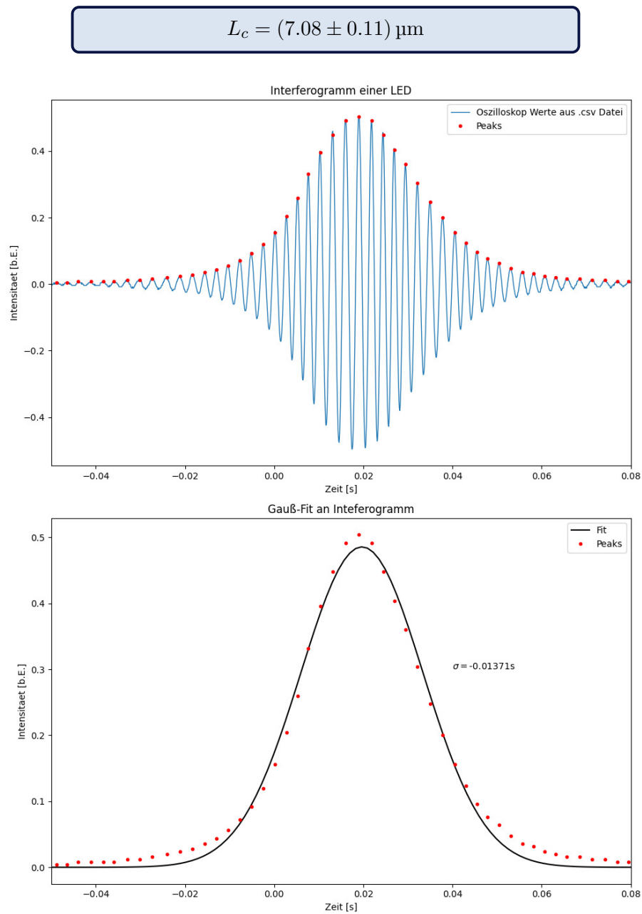
Abb. 3.2: an das Bild der aufgenommenen Oszilloskopdaten wurde eine Gaußkurve gefittet
