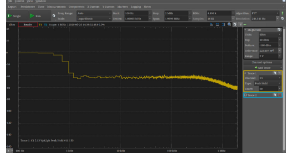
(b) Spektrum bei R = 30 \text{ k}\Omega
