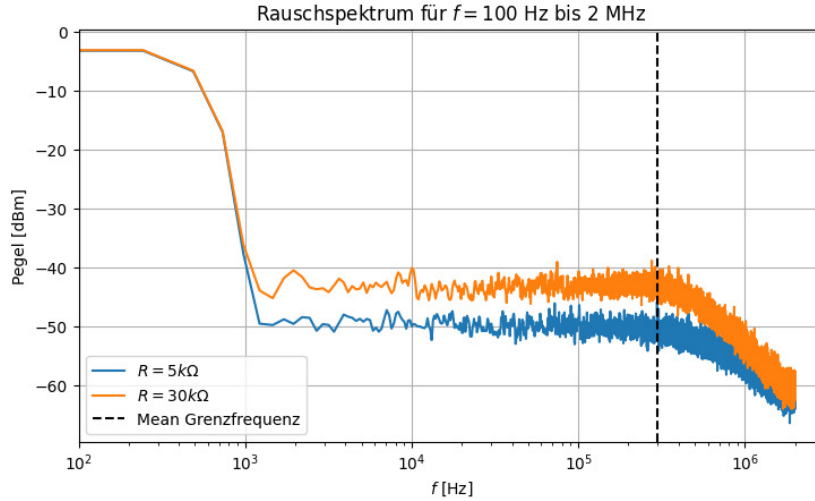
Abb. 3.2: Rauschpegel Plot (5, 30) k \Omega
