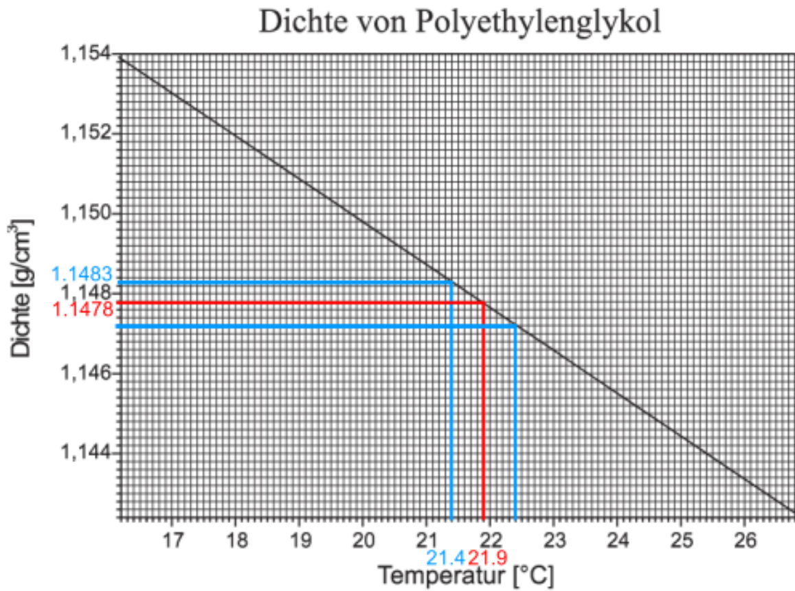
Abb. B.1: Dichte von Polyethylenglykol 1
