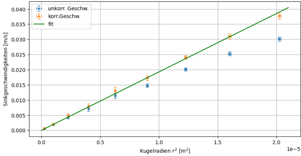
Abb. 3.1: uncorr. und korr. Sinkgeschwindigkeiten der Kugeln mit Fitgerade
