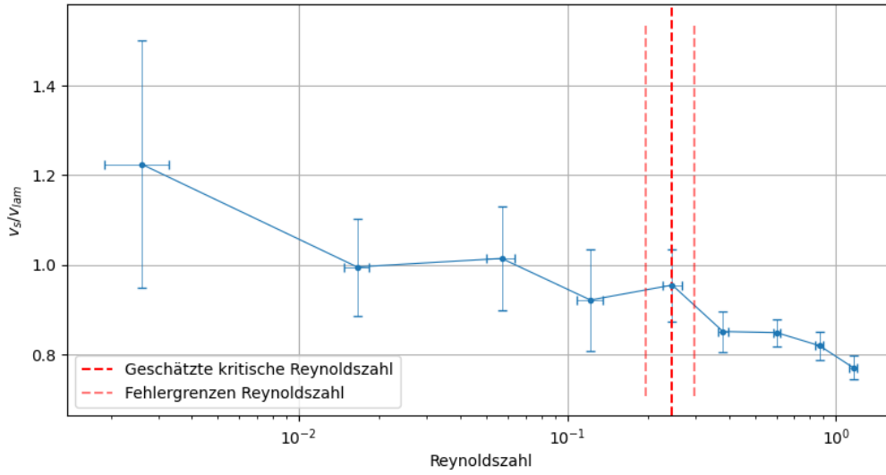
Abb. 3.3: verzweifelter Extrahieren der Grenze von laminarer zu turbulenter Strömung
