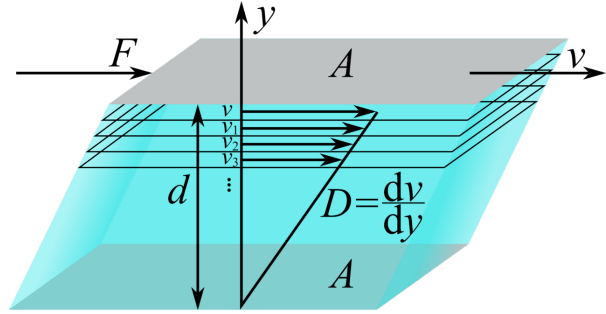
Abb. 1.2: schichtweises Bewegen der Flüssigkeit Richtung Kraft F 4
