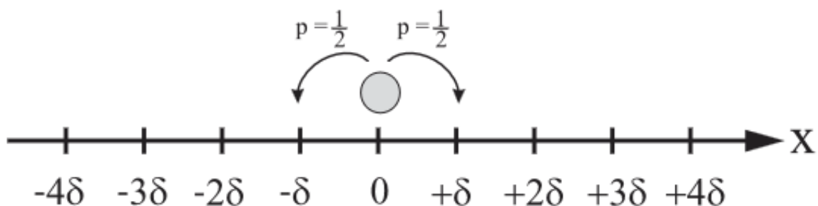
Abb. 1.2: Eindimensionaler Random-Walk 1
