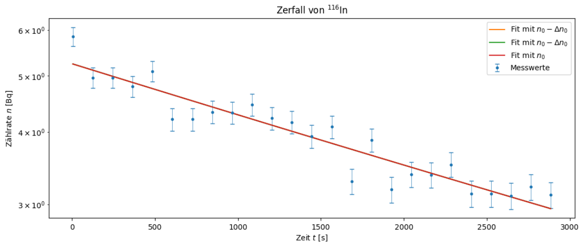
Abb. 3.2: Fit der Zerfallsfunktion für Indiumisotope
