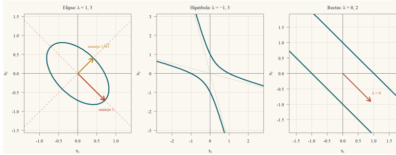
Figura 1: Los tres casos de x'Ax = 1 en el plano. Izquierda: A = \begin{pmatrix} 2 & 1 \\ 1 & 2 \end{pmatrix} , valores propios 1 y 3: elipse con semiejes 1 (a lo largo de (1, -1) ) y 1/\sqrt{3} (a lo largo de (1, 1) ). Centro: A = \begin{pmatrix} 1 & 2 \\ 2 & 1 \end{pmatrix} , valores propios -1 y 3: hipérbola ( 3y_1^2 - y_2^2 = 1 ). Derecha: A = \begin{pmatrix} 1 & 1 \\ 1 & 1 \end{pmatrix} , valores propios 0 y 2: las rectas x + y = \pm 1 , porque x'Ax = (x + y)^2 .
