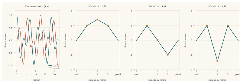
Figura 5: Izquierda: dos masas con x(0) = (1, 0) : la energía se intercambia entre ellas. Tres modos de tres masas: el patrón de desplazamientos de cada modo normal (las paredes en los extremos) y su frecuencia \omega .
