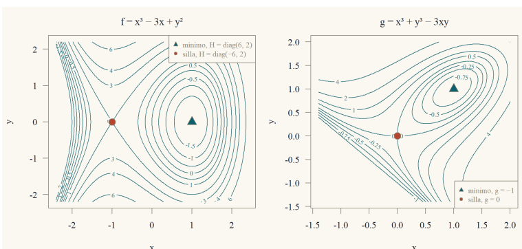
Figura 4: Curvas de nivel de dos funciones con sus puntos críticos.
