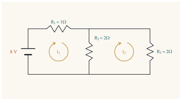
Figura 1: Un circuito de dos mallas. Las flechas circulares son las corrientes de malla i_1 e i_2 , que suponemos en el sentido de las agujas del reloj.
