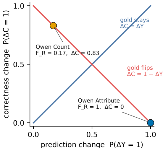
(a) Lemma 4 geometry
